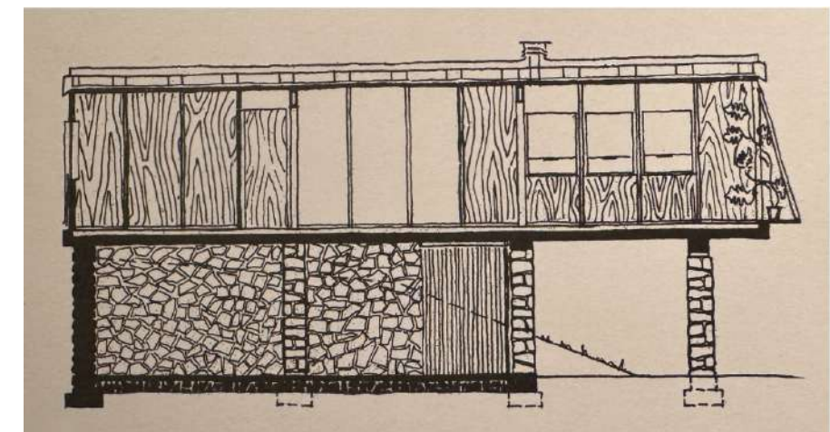
© Coupe longitudinale sur une maison à portique (D.R) © Longitudinal view of a porticoed house (R.R)
